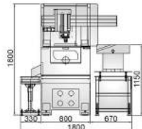
震動盤送料
